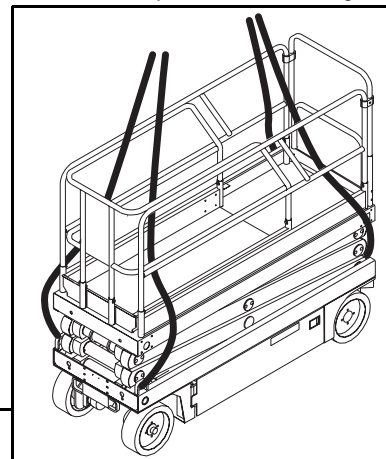
Figure 6: Fije las correas de la grúa
