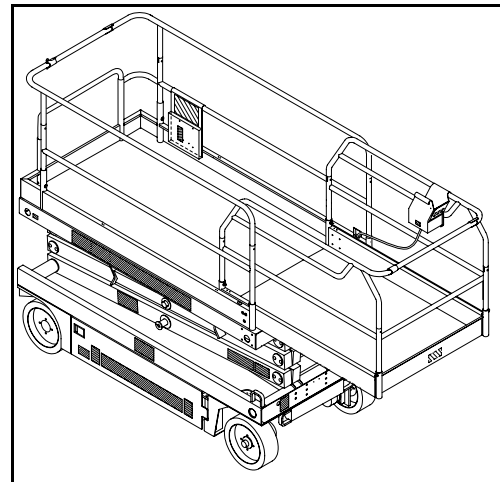
Abbildung 4: Plattformverlängerung
