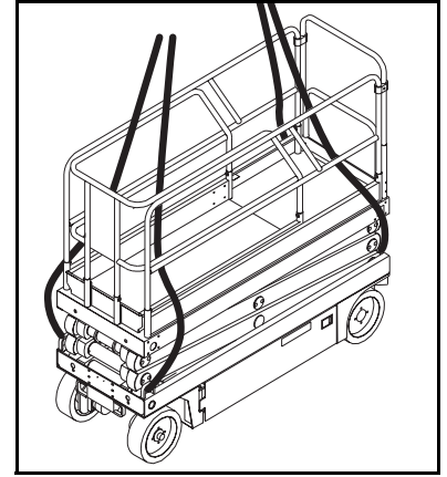
Figura 6: Cinghie di fissaggio per gru
