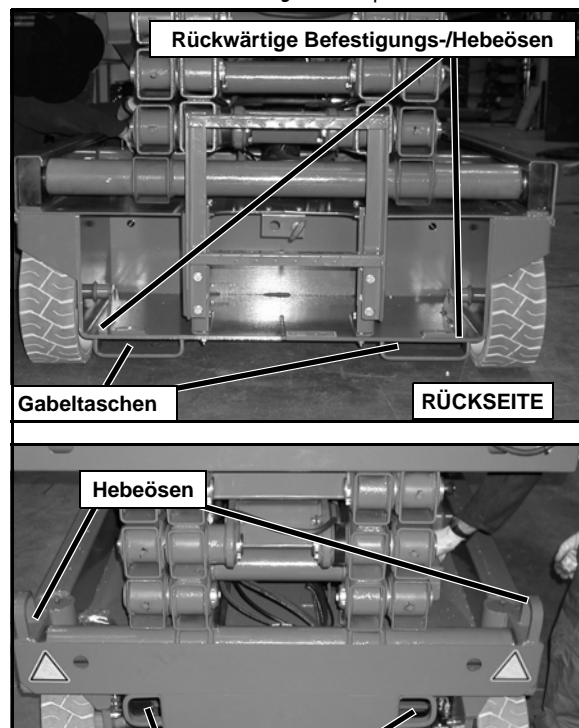
Abbildung 7: Transport der Arbeitsbühne
