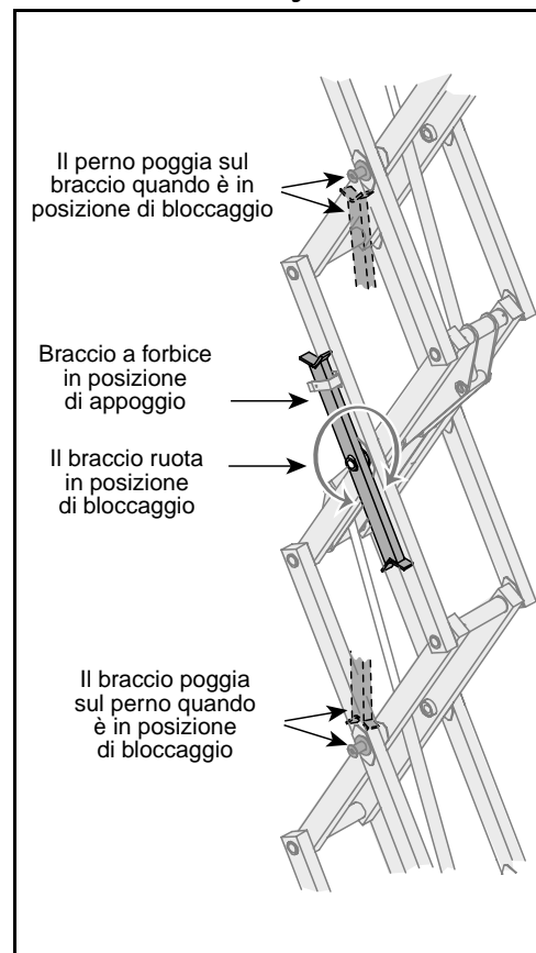
Figura 8: Braccio a forbice
