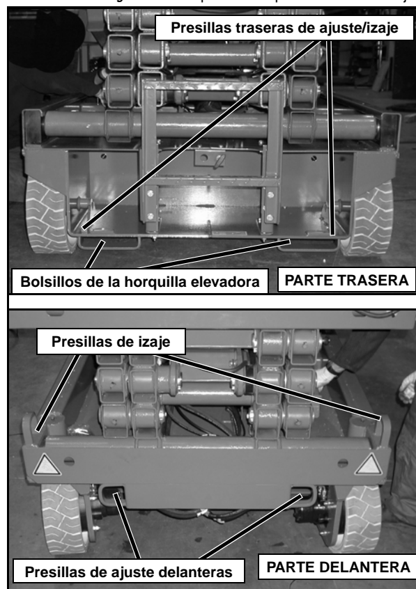
Figure 7: Transporte de la plataforma de trabajo
