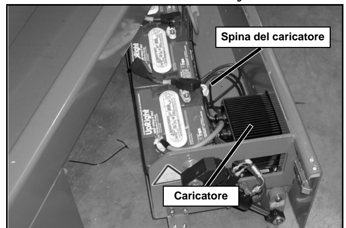
Figura 9: Caricabatterie
