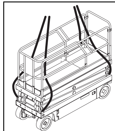
Abbildung 6: Sichern Sie die Krangurte.
