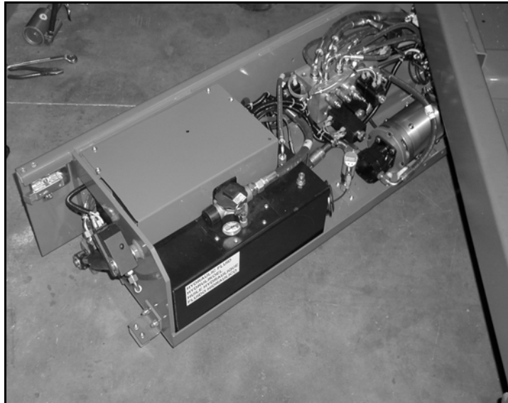
Figure 3: Tanque hidráulico
